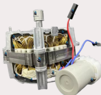
Motor WEG 127V Modelo Arno Cod.000127
