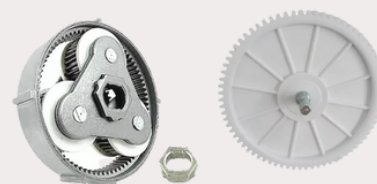
Planetário Arno C/ Engrenagem 74 Dentes E Bucha Cod. 830991
