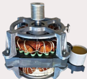
Motor WEG 220V Modelo Suggar Cod. 000220
