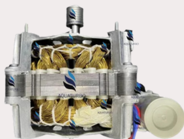
Motor WEG 127V Modelo Britania Cod. 000127
