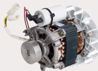
Motor Lavadora De Roupas Plus Mueller 1/5cv 220V Cod. 605005
