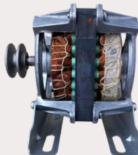
Motor De Tanquinho Libell, Lave Mais, Fioreta, Cimento 220V Cod. 191181
