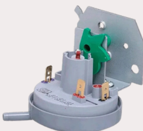
Pressostato 4 Niveis Lavadora Brastemp 326050133 Bwl09/07 Cod. 050133
