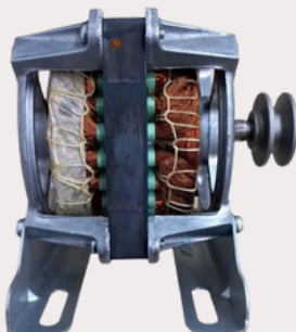
Motor De Tanquinho Libell, Lave Mais, Fioreta, Cimento 127V Cod. 351334
